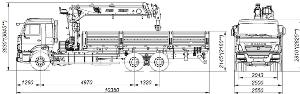
Размеры для автомобиля снаряженной массы: * - с шинами 11.00 R22,5/ ** - с шинами 11.00 R20
